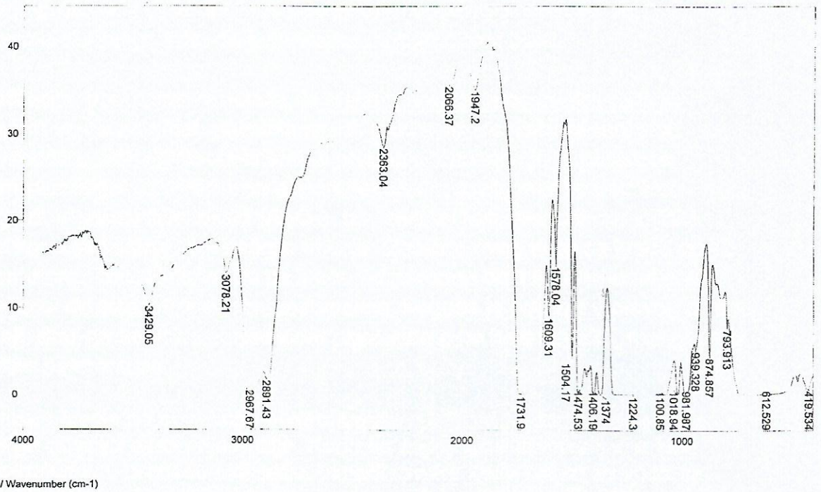
Slika 3b. FTIR spektrograf uzoraka proizvoda (III)
